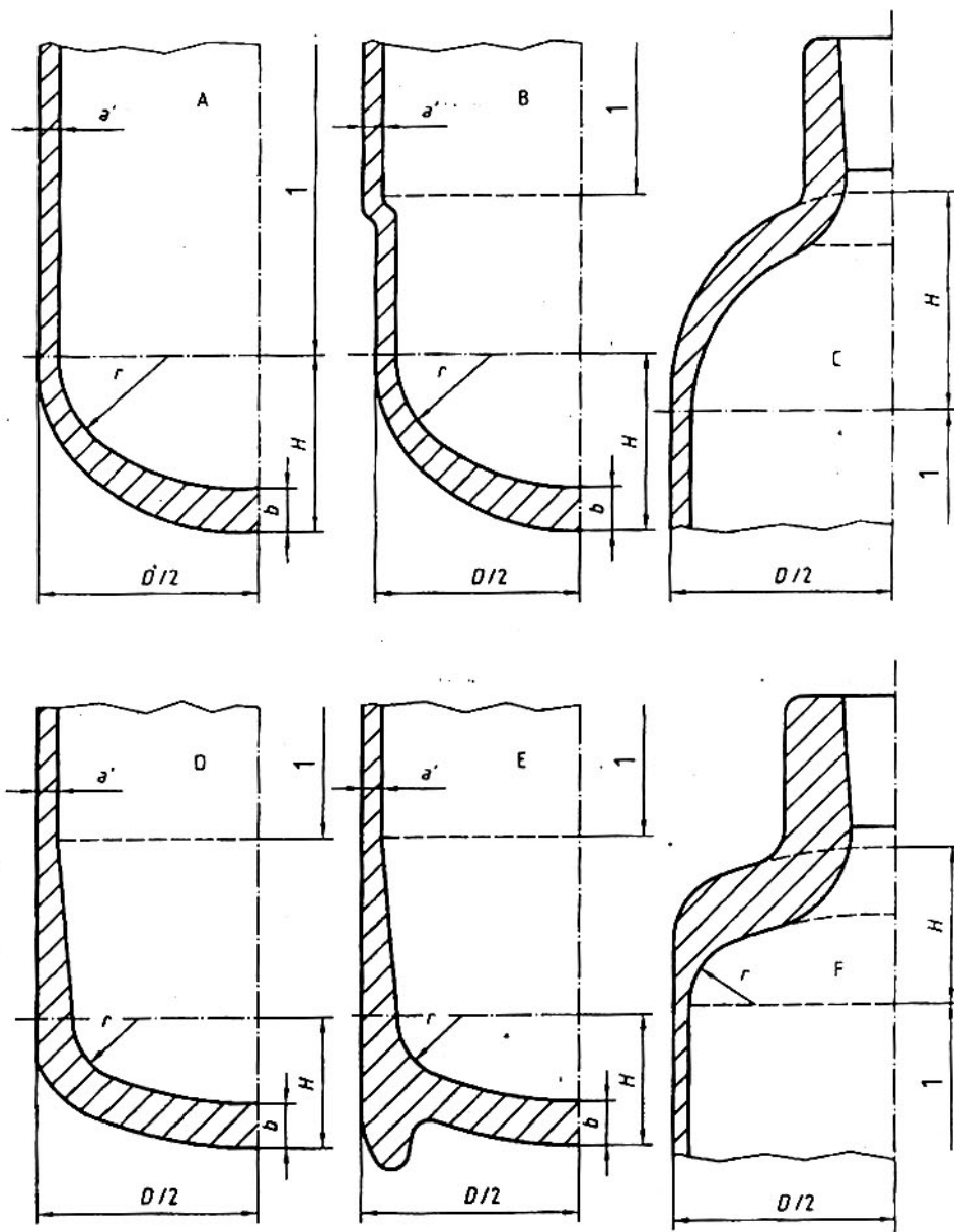
Hình 1 – Các đỉnh và đáy lõi điển hình của đai
