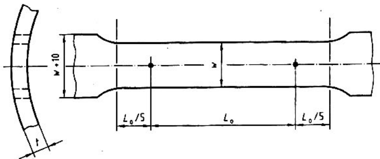
Hình 5 – Mẫu thử kéo
