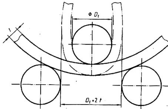
Hình 6 – Minh họa phép thử uốn
