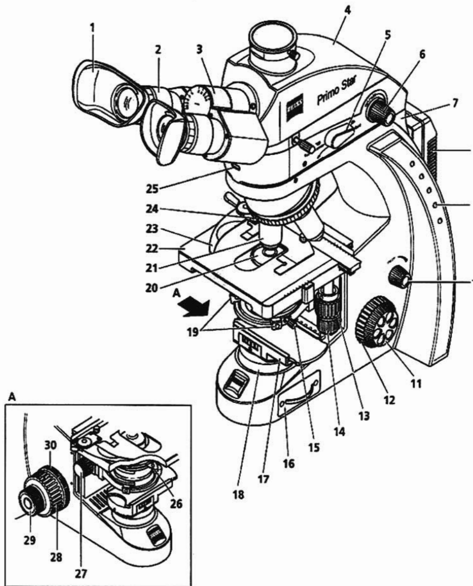
Fig. 15 Controls of Primo Star ILED
