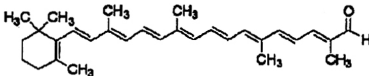
Hình 1 – Công thức cấu tạo của all-trans - \beta -apo-8'-carotenal (hợp chất chính)
