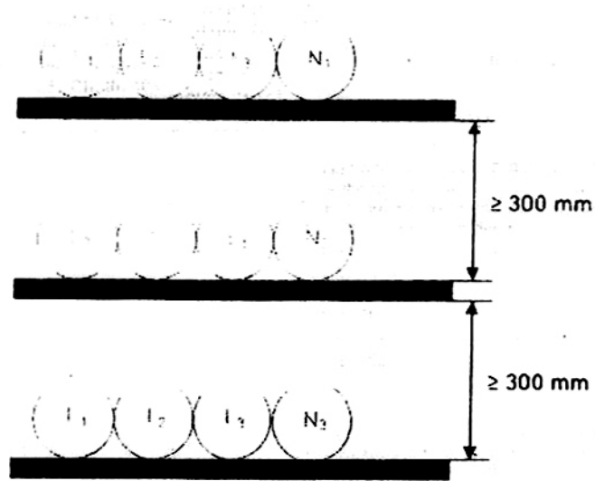
Hình H.52.5 – Cấu hình cụ thể đối với 9 cáp một lõi song song dây này đặt cao hơn dây kia (xem 523.7)
