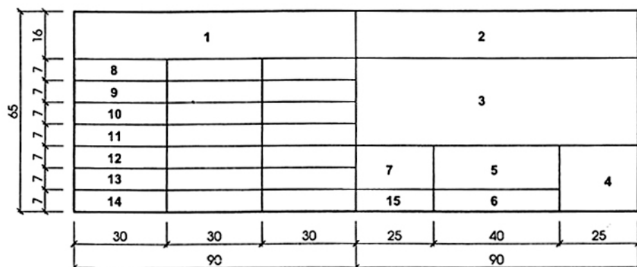
Hình 2 – Kích thước, nội dung và cách trình bày khung tên
