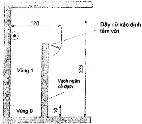
2) Hình chiếu cạnh (có vách ngăn cố định và bán kính xác định khoảng cách tối thiểu từ đầu phía trên của vách ngăn
