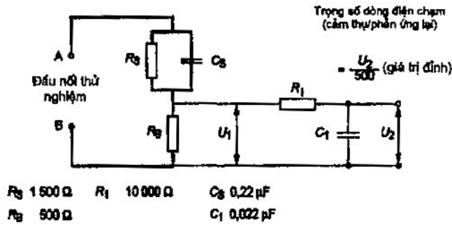
Hình G.2 – Mạng đo, trọng số dòng điện chạm cảm thụ hoặc phản ứng lại (đối với tất cả đèn điện cấp II và đèn điện cố định cấp I)
