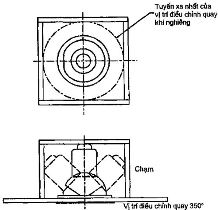
Hình D.2 – Kích cỡ hộp thử nghiệm đúng (trần cách điện) đối với đèn điện điều chỉnh được
