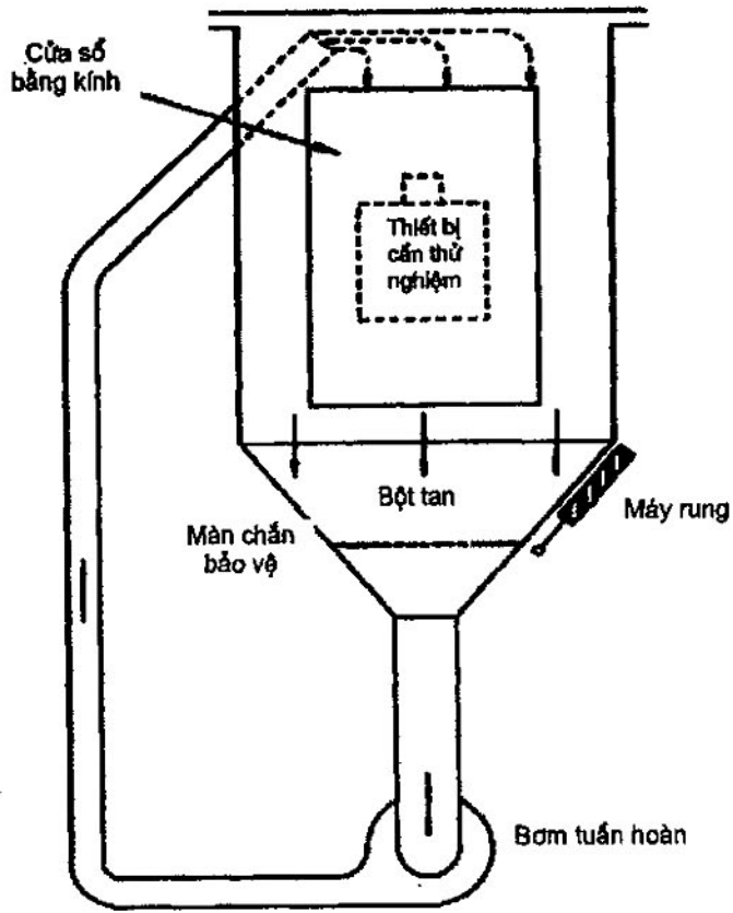
Hình 6 – Trang bị để thử bảo vệ chống bụi
