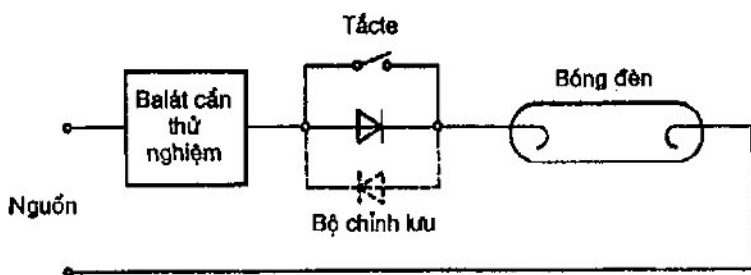
Hình C.2 – Mạch điện dùng để thử nghiệm hiệu ứng chỉnh lưu (balát dùng cho các bóng đèn một chân)
