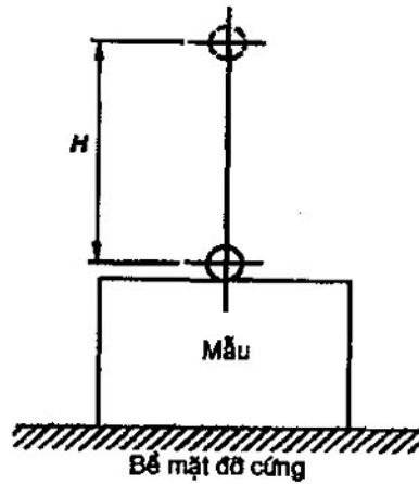
Hình 21 – Thiết bị để thử nghiệm và đập bằng viên bi
