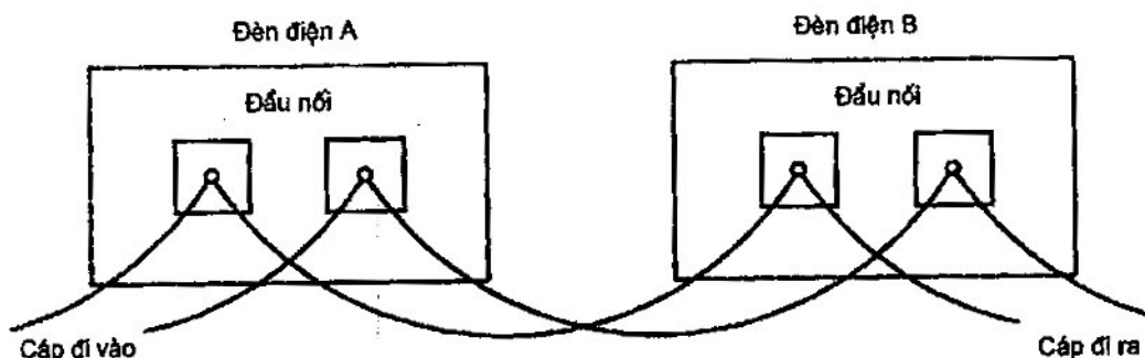
Hình 20A – Minh họa thuật ngữ "đi dây nguồn song song"
