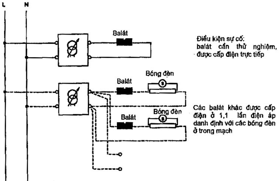
Hình 32 – Mạch điện thử nghiệm dùng cho đèn điện có lắp bóng đèn huỳnh quang \leq 70 W
