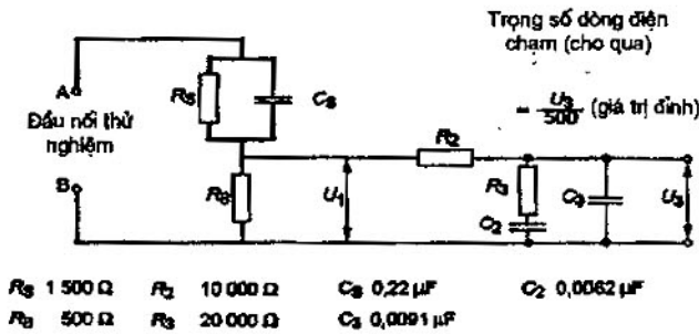
Hình G.3 – Mạng đo, trọng số dòng điện chạm cho qua
