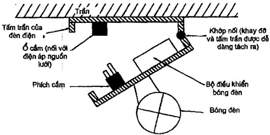
Hình 31 – Hệ thống tiếp điểm điện cơ có mối nối kiểu phích cắm/ổ cắm
