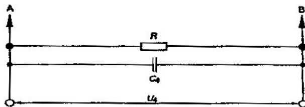
Hình G.3 – Mạng đo, trọng số dòng điện chạm cho qua
