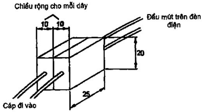
Hình 2 – Bố trí khối đầu nối để thử nghiệm lắp đặt đối với đèn điện có các đầu nút
