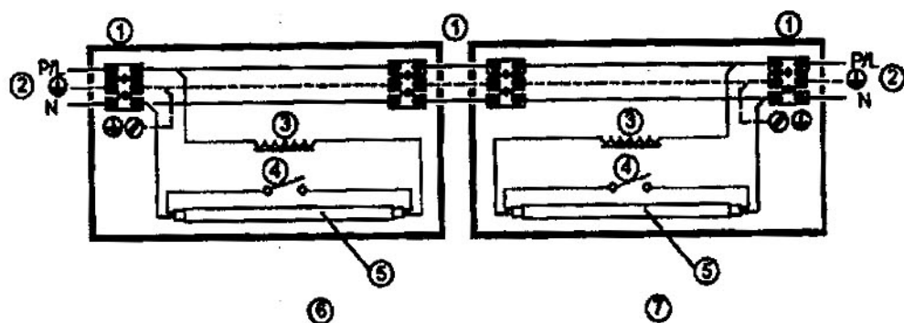
Hình 20A – Minh họa thuật ngữ "đi dây nguồn song song"
