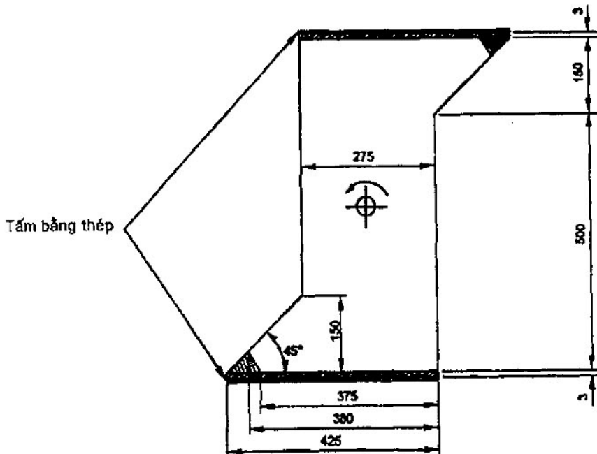
Hình 24 – Minh họa phép đo chiều dài đường rò và khe hở không khí ở đầu nối nguồn Kích thước tính bằng milimét.
