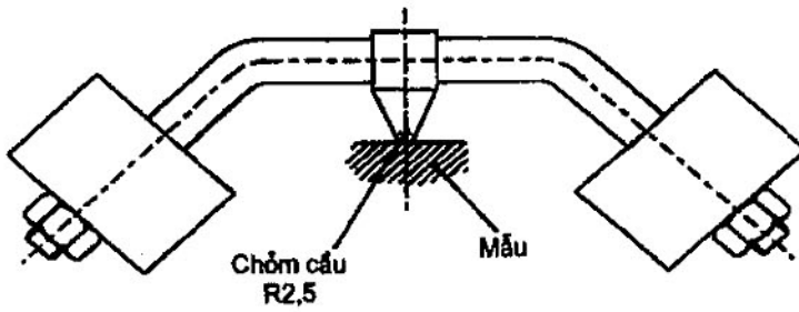
Hình 10 – Thiết bị ép viên bi
