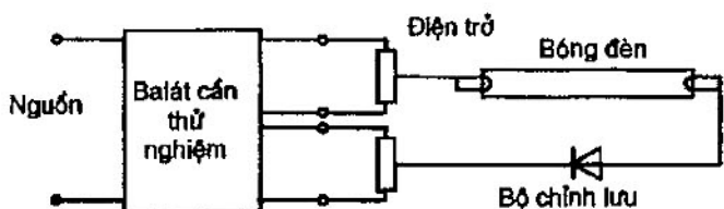
Hình C.1 – Mạch điện dùng để thử nghiệm hiệu ứng chỉnh lưu (chỉ cho một số balát điện dung không có tắc te)
