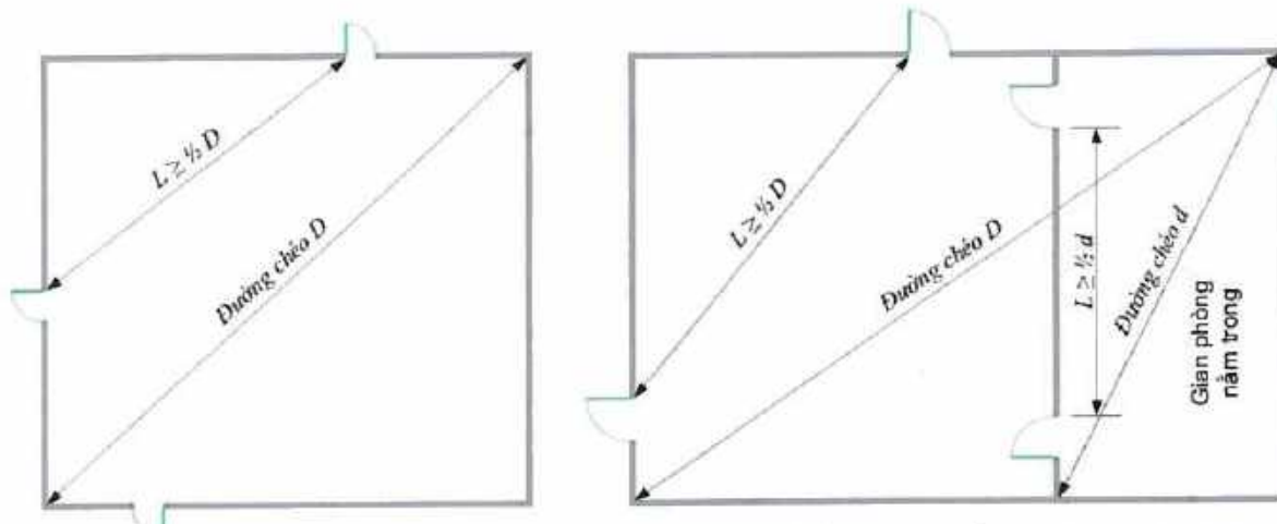
b) Minh họa về bố trí phân tán lối ra thoát nạn của các gian phòng nằm trong một gian phòng khác hoặc một phần nhà, một tầng nhà
